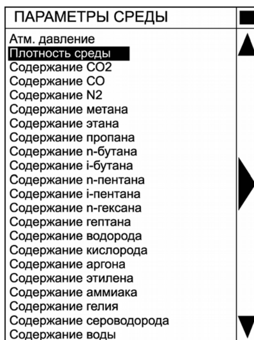
Рисунок 15 — Меню «ПАРАМЕТРЫ СРЕДЫ»
