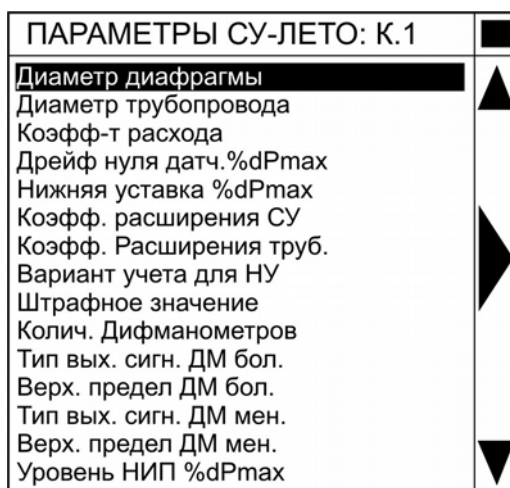
Рисунок 20 — Меню «НАСТРОЙКА СУ-ЗИМА (ЛЕТО)»
