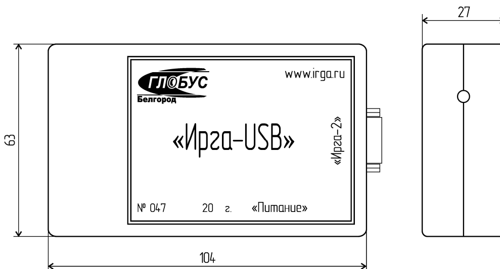
Рисунок 1 – Габаритный чертеж адаптера
